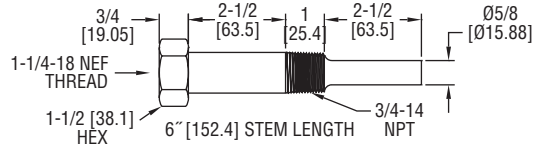
Lag Thermowell
